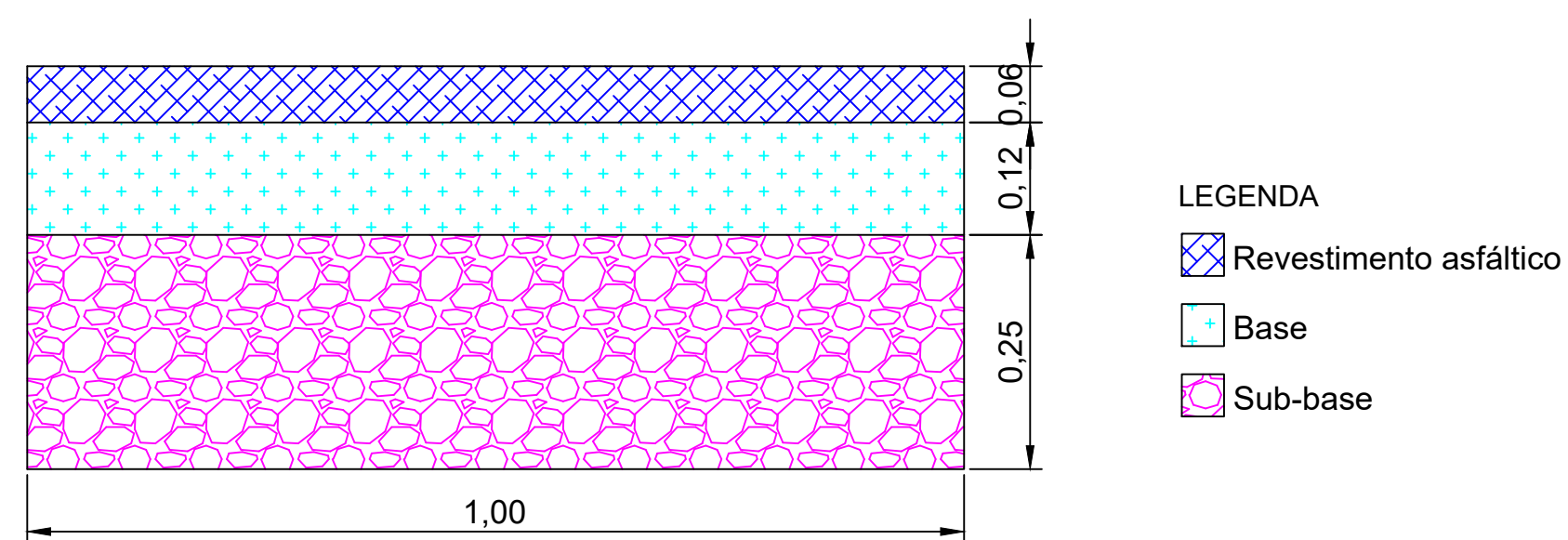
Perfil pavimento a executar nos locais com canteiro a retirar
